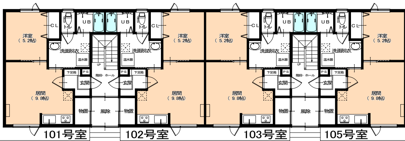
1階平面図
